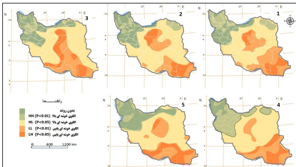
شکل (۳). الگوهای فضایی طول دوره‌های بارشی ایران بر اساس آماره موران محلی انسلین (LMI) (۱ دوره اول: ۱۹۹۵-۱۹۹۹، ۲ دوره دوم: ۲۰۰۰-۱۹۹۶، ۳ دوره سوم: ۲۰۰۵-۲۰۰۱، ۴ دوره چهارم: ۲۰۱۰-۲۰۰۶، ۵ دوره پنجم: ۲۰۱۵-۲۰۱۱) منبع: نگارندگان مقاله
