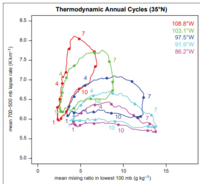
شکل (۱). چرخه سالانه آهنگ افت دمای لایه‌های میانی و رطوبت در سپهر ۵۰۰-۷۰۰ هکتوپاسکال
