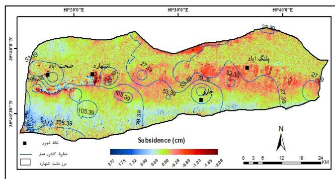
شکل (۳۵). هم پوشانی نقشه فرونشست (۲۰۲۳ - ۲۰۲۲) با میانگین تراز عمق آب زیرزمینی (۲۰۲۲)
