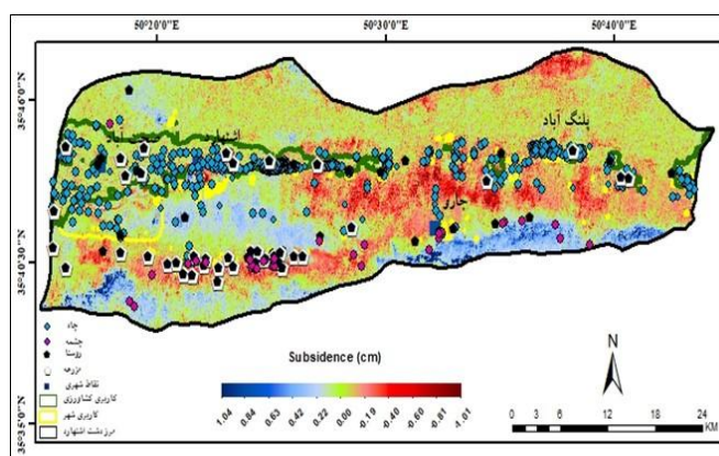
شکل (۱۲). هم‌پوشانی نقشه کاربری، منابع آب (چشمه و چاه)، مزارع و آبادی منطقه مورد مطالعه بر روی نقشه میانگین فرونشست بازه هفت‌ساله (۲۰۲۳ - ۲۰۱۷)
