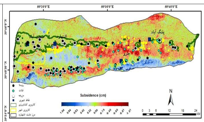
شکل (۱۱). هم‌پوشانی نقشه کاربری، منابع آب (قنات)، مزارع و آبادی منطقه مورد مطالعه بر روی نقشه میانگین فرونشست بازه هفت ساله (۲۰۲۳ - ۲۰۱۷)
