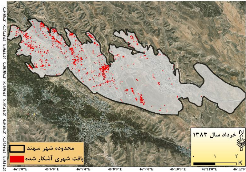
خرومی الگوریتم طبقه‌بندی نظارت شده MLC برای خرداد سال ۲۰۰۵ - سنجنده TM لندست ۵
