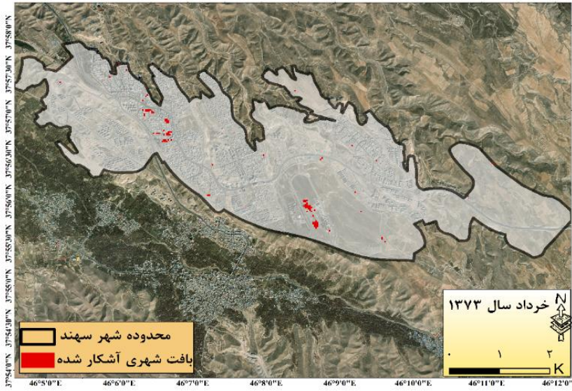
خرومی الگوریتم طبقه‌بندی نظارت شده MLC برای خرداد سال ۱۹۹۵ - سنجنده TM لندست ۵
