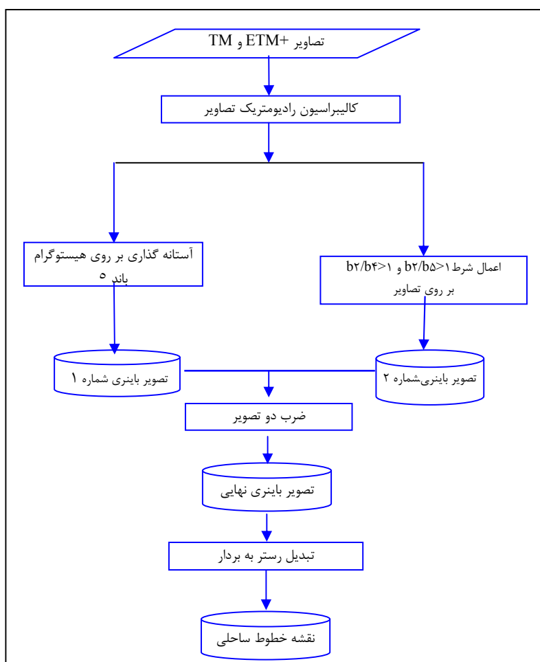
شکل ۱؛ فلوجارت استخراج خط ساحلی از تصاویر TM ETM+
