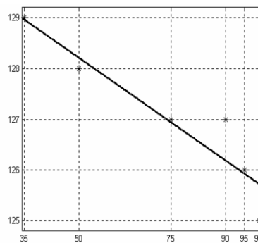
احتمال (ب)
