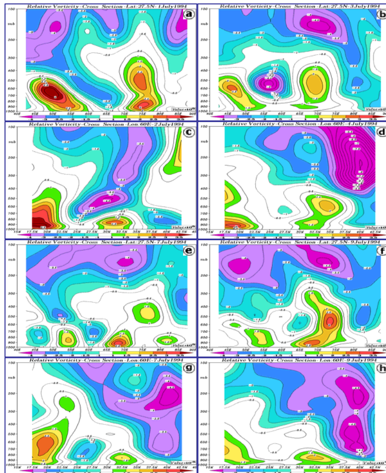
شکل ۷. نیمرخ قائم تاوایی نسبی با استفاده از داده‌های ۱۲ تراز فشاری، برحسب 10^{-5} s^{-1} برای روزهای دهه اول جولای ۱۹۹۴ (a, b, e) و نیمرخ قائم در امتداد عرض ۲۷٫۵ درجه شمالی و (c, d, g, h) نیمرخ قائم در امتداد طول ۶۰ درجه شرقی. در شکل‌ها از نشان‌دادن مقادیر تاوایی بین 10^{-5} s^{-1} و 10^{-5} s^{-1} صرف‌نظر شده است.
