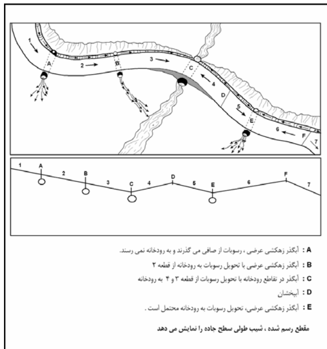
شکل ۲- زهکشی سطح جاده و عوارض زهکشی
