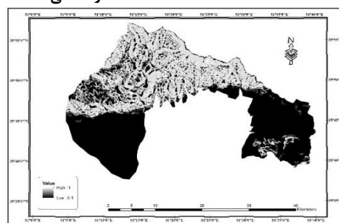
شکل ۷. فازی سازی طبقات شیب.
