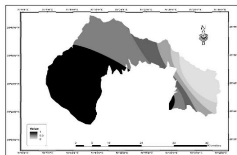
شکل ۹. فازی سازی طبقات بارش سالانه.
