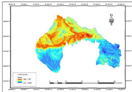
شکل ۲۱. نقشه‌ی پهنه‌بندی خطر زمین لغزش با عملکرد جمع فازی.
