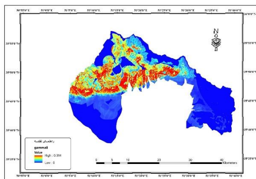
شکل ۲۳. نقشه‌ی پهنه‌بندی خطر زمین لغزش با عملکرد گامای فازی ۰/۸.
