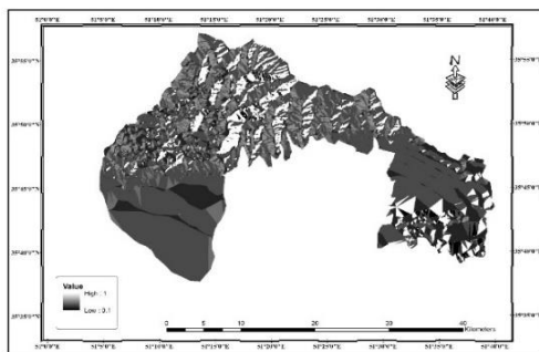
شکل ۸. فازی سازی طبقات جهات شیب.
