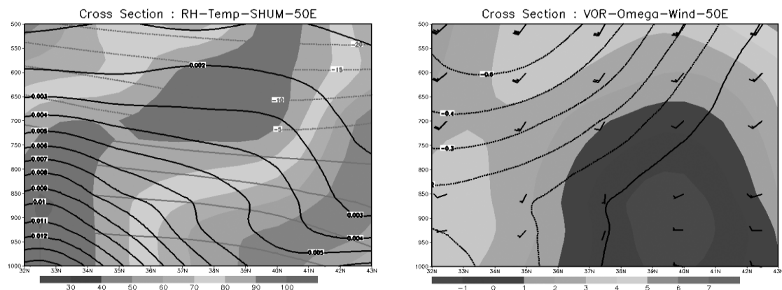
شکل ۲۵: برش قائم میدان تاوایی نسبی (بر ثانیه رنگی شده)، برش قائم میدان سرعت قائم (بر حسب متر بر ثانیه خطوط هم‌مقدار مشکی رنگ)، برش قائم میدان باد (بر حسب متر بر ثانیه) برای ساعت ۰۹ گرینویچ روز ۱۳ دسامبر ۲۰۱۰.
