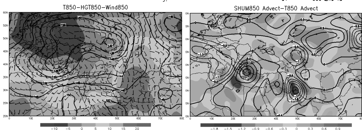
شکل ۲۴: میدان تاوایی نسبی (مقادیر رنگی شده بر حسب عکس ثانیه)، ارتفاع ژئوپتانسیلی (خطوط مشکی بر حسب دکامتر) میدان دما (خطوط رنگی بر حسب درجه‌ی سلسیوس) در تراز ۵۰۰ هکتوپاسکالی برای ساعت ۱۲ گرینویچ روز ۱۳ دسامبر ۲۰۱۰.
