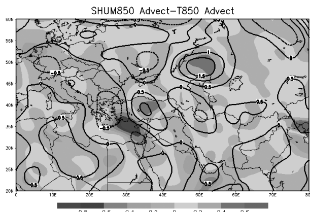
شکل ۱۳: فرارفت رطوبت ویژه (مقادیر رنگی شده بر حسب درجه‌ی سلسیوس بر ثانیه) و فرارفت دما (خطوط هم‌مقدار) در تراز ۸۵۰ هکتوپاسکال برای ساعت ۰۶.
