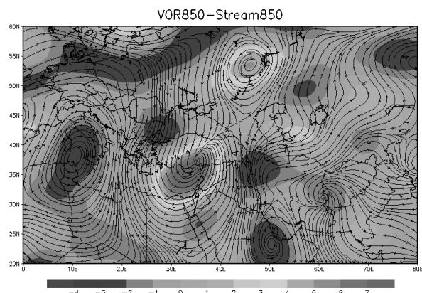
شکل ۳: میدان تاوایی نسبی (مقادیر رنگی شده بر حسب عکس ثانیه) و جریان تراز ۸۵۰ هکتوپاسکالی (خطوط پیوسته) برای ساعت ۱۲ گرینویچ روز ۲۹ ژانویه ۲۰۰۸.
