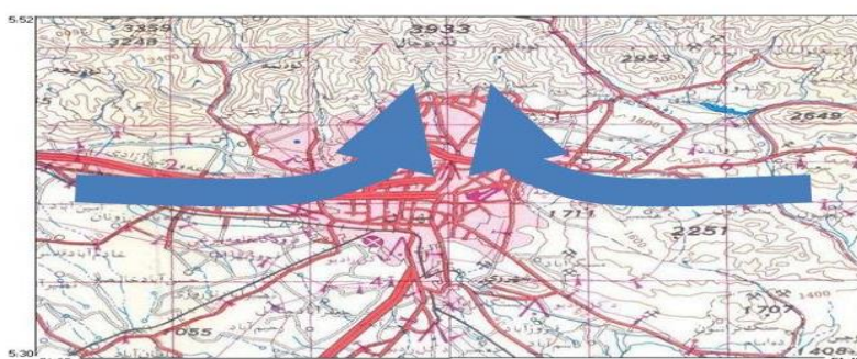
شکل ۱۱: جریان هوا در ترازهای پایینی از اطراف تهران به سمت مرکز (تحت تأثیر کم‌فشار تشکیل شده ناشی از
