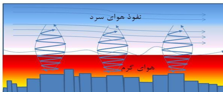
شکل ۱۰. تشدید اختلاف دما بین سطح زمین و ترازهای بالایی سبب افزایش حرکات قائم شده
