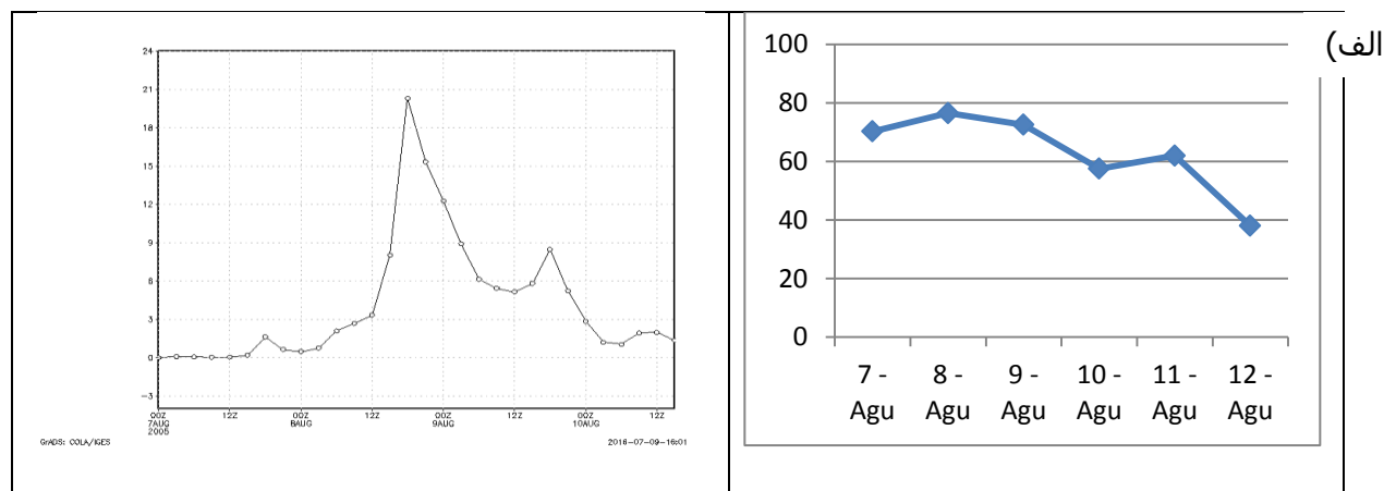
شکل ۹: غلظت گردوغبار کل ( \frac{\mu g}{kg(dry\ air)} ) در روزهای ۱۶ تا ۱۹ مرداد ماه سال ۱۳۸۴ در شهر تبریز (الف) میانگیری شده از داده‌های ساعتی سازمان محیط زیست کشور (ب) اجرای مدل WRF-Chem
