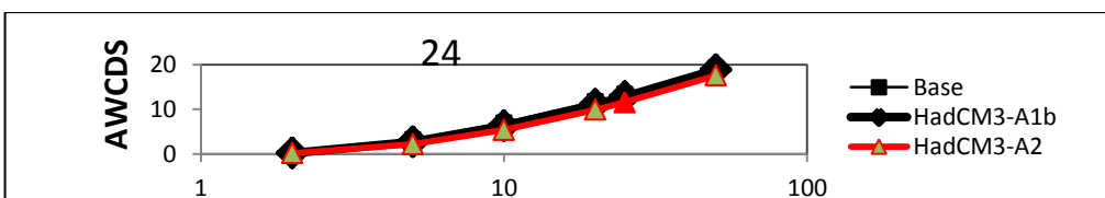
شکل ۱۲: شدت تجمعی خشکسالی به ترتیب از بالا به پایین برای برای تداوم زمانی ۳، ۱۲ و ۲۴ ماهه در دوره مشاهداتی، A۱B و A۲ و برای دوره برگشت ۲ تا ۵۰ سال برای مناطق مرکزی ایران
