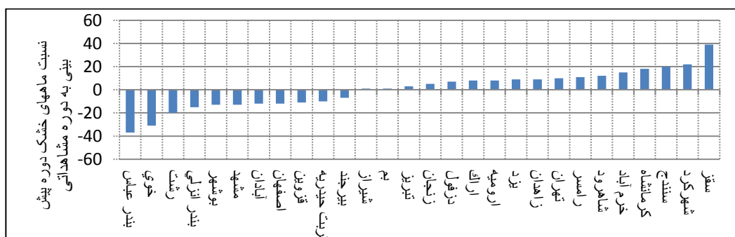
شکل ۵: نسبت فراوانی خشکسالی ایستگاههای منتخب دوره مشاهداتی و دوره ۲۰۱۱-۲۰۴۰ براساس
