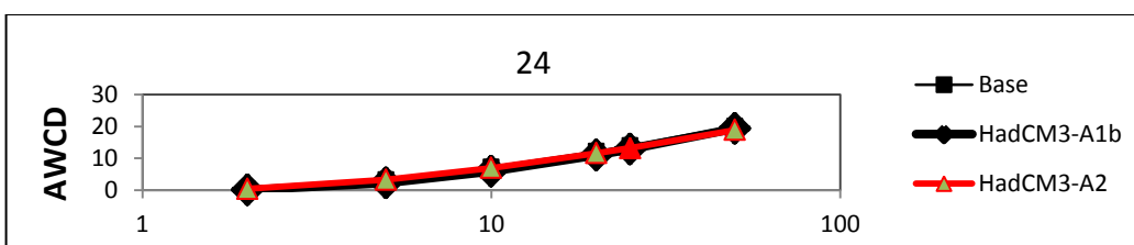
شکل ۹: شدت تجمعی خشکسالی به ترتیب از بالا به پایین برای تداوم زمانی ۳، ۱۲ و ۲۴ ماهه در دوره مشاهداتی، A1B و A2 برای دوره برگشت ۲ تا ۵۰ سال برای غرب کشور
