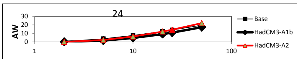
شکل ۱۳: شدت تجمعی خشکسالی به ترتیب از بالا به پایین برای برای تداوم زمانی ۳، ۱۲ و ۲۴ ماهه در دوره مشاهداتی، A۱B و A۲ و برای دوره برگشت ۲ تا ۵۰ سال برای مناطق جنوبی ایران
