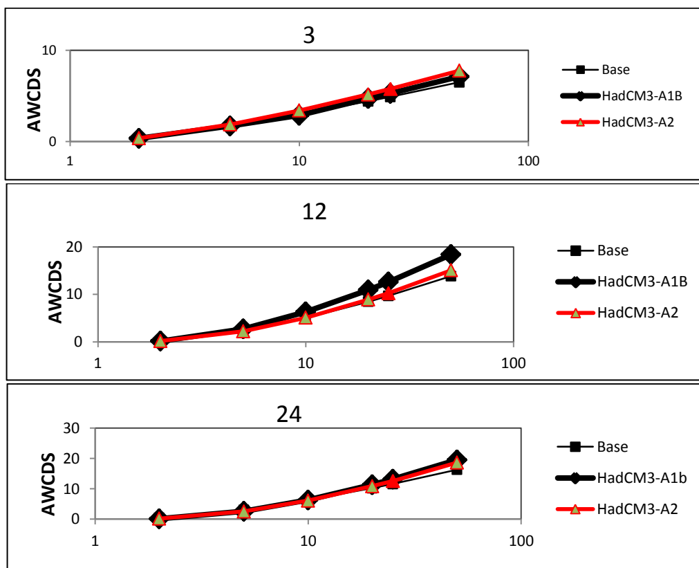
شکل ۱۶: شدت تجمعی خشکسالی به ترتیب از بالا به پایین برای تداوم زمانی ۳، ۱۲ و ۲۴ ماهه در دوره مشاهداتی، A1B و A2 و برای دوره برگشت ۲ تا ۵۰ سال برای جنوب شرق ایران
