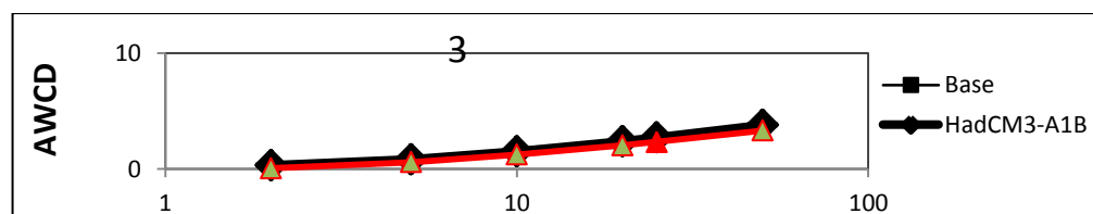
شکل ۱۲: شدت تجمعی خشکسالی به ترتیب از بالا به پایین برای برای تداوم زمانی ۳، ۱۲ و ۲۴ ماهه در دوره مشاهداتی، A۱B و A۲ و برای دوره برگشت ۲ تا ۵۰ سال برای مناطق مرکزی ایران
