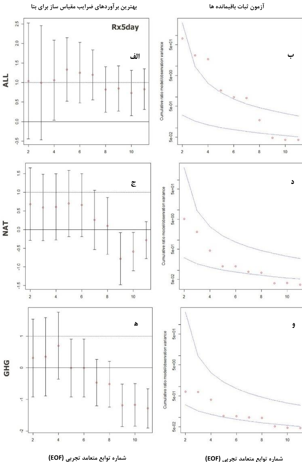
شماره توابع متعامد تجربی (EOF) الف بهترین ضرایب مقیاس ساز برای سیگنال های ALL, NAT, GHG مربوط به Rx5day شماره توابع متعامد تجربی (EOF) ب و نتایج آزمون ثبات باقیمانده ها (کادر سمت راست)
