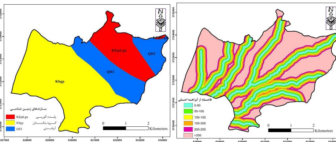
شکل ۵: نقشه طبقه‌بندی شده فاصله از آب‌راه اصلی
