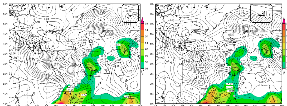
شکل ۷. نقشه‌های ترکیبی مجموع رطوبت (۵۰۰-۷۰۰) و امگا برحسب پاسکال بر ثانیه در ترازهای الف: ۷۰۰، ب: ۵۰۰
