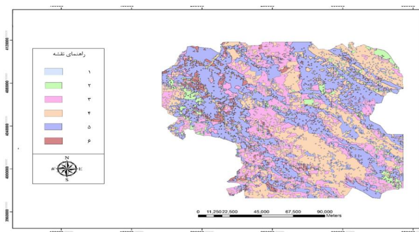
شکل ۱۱: پهنه بندی مکان بهینه دفن پسماند های استان زنجان
