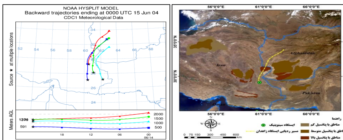
شکل ۷- رهگیری باد بهنگام وقوع گرد و غبار ۱۷/۰۶/۲۰۰۴-۱۵
