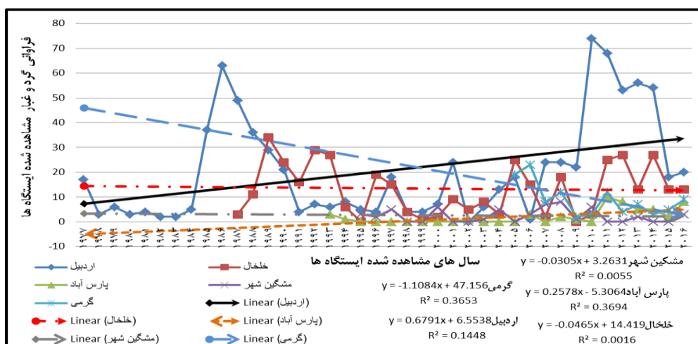
شکل ۷: نمودار فرآوانی گرد و غبار سالانه در سال‌های مشاهده شده
