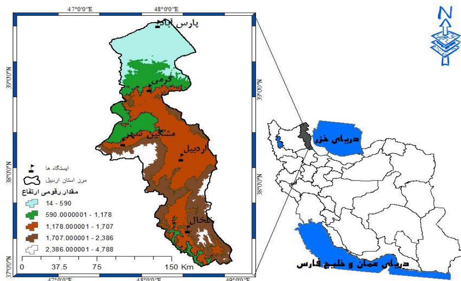
شکل ۱: موقعیت منطقه مورد مطالعه در ایران
