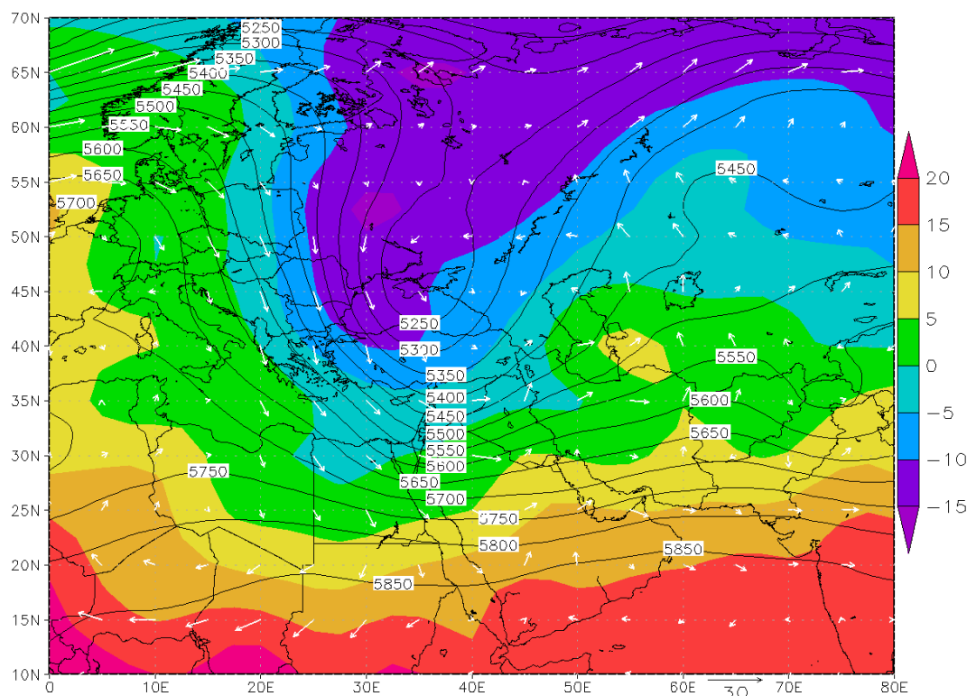
شکل ۱۰: نقشه ترکیبی ارتفاع ژ.پ تراز ۵۰۰ ه.پ (کنطور)، دما (°C) (پهنه رنگی) و بردارهای سمت و سرعت باد (m/s) تراز ۸۵۰ ه.پ تاریخ ۱۹۹۲/۰۲/۰۷
