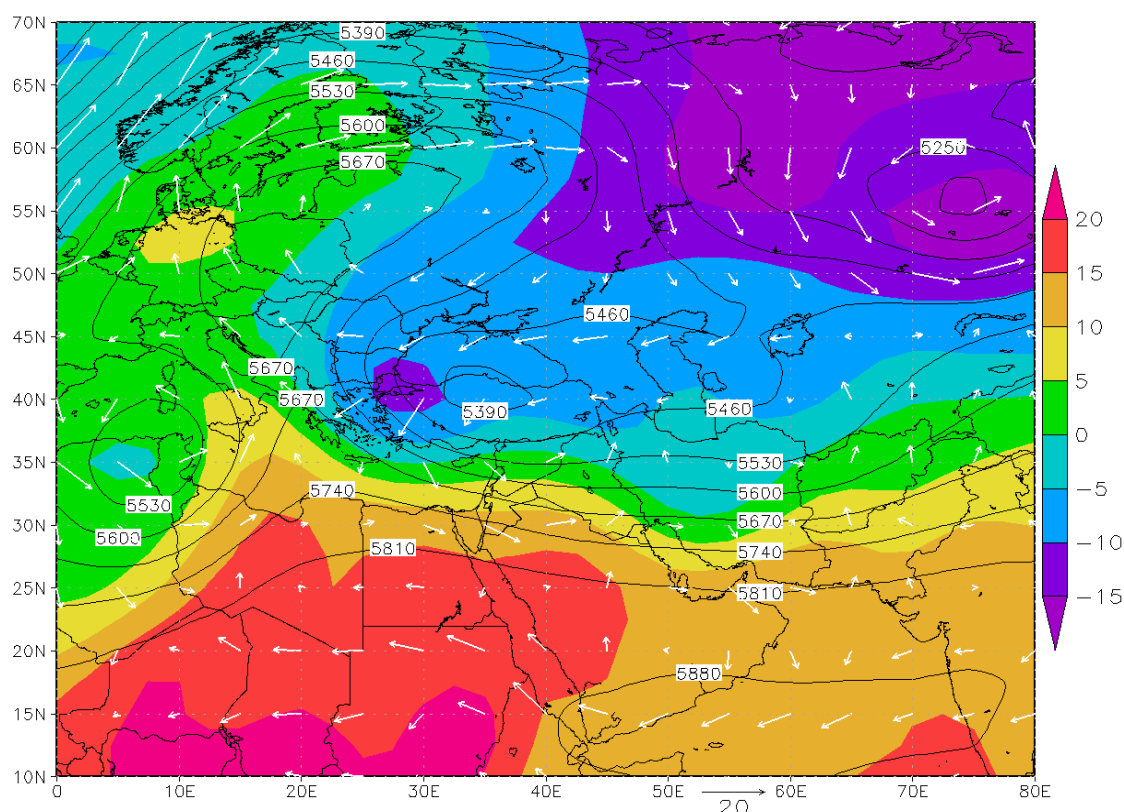
شکل ۱۲: نقشه ترکیبی ارتفاع ژ.پ تراز ۵۰۰ ه.پ (کنتور)، دما (C°) (پهنه رنگی) و بردارهای سمت و سرعت باد (m/s) تراز ۸۵۰ ه.پ تاریخ ۱۳۹۰/۱۲/۲۵.
