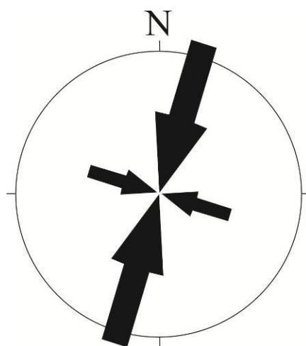
شکل ۱۱. موقعیت تنش‌های اصلی بیشینه (۰۱۷/۰۲) و میانه (۰۱۷/۰۰) به دست آمده از کل داده‌های گسلی در منطقه مورد مطالعه پس از چرخش داده‌ها. (محور تنش اصلی کمینه قائم است.)
