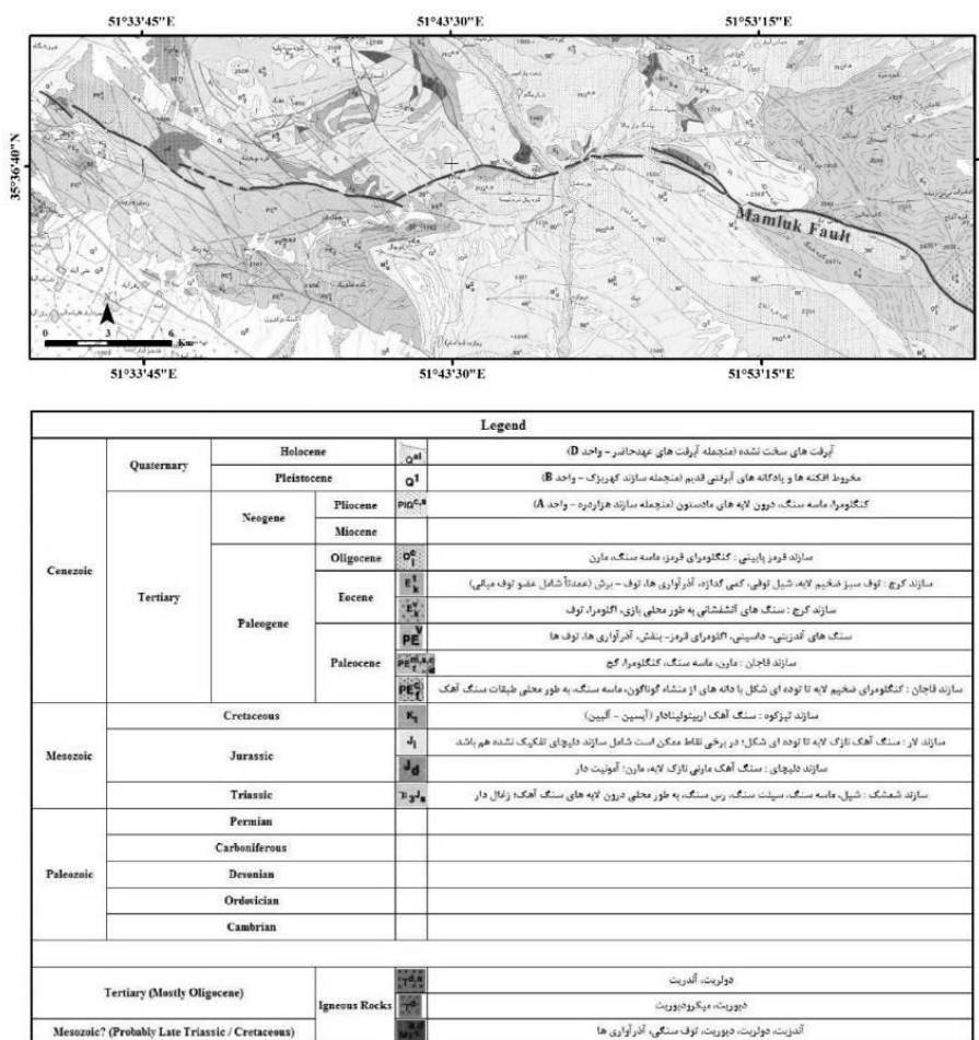
شکل ۳. گسل ماملوک و قصر فیروزه (برگرفته از نقشه زمین‌شناسی ۱:۱۰۰،۰۰۰ شرق تهران، سازمان زمین‌شناسی و اکتشافات معدنی کشور - دلباخ و وحدتی، ۱۹۶۴ و بربریان و همکاران، ۱۳۷۱)
