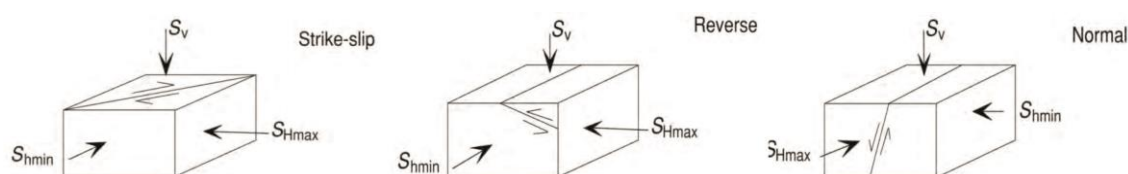
شکل ۹: تصویر شماتیک شکل گیری گسل ها برپایه تئوری آندرسون
