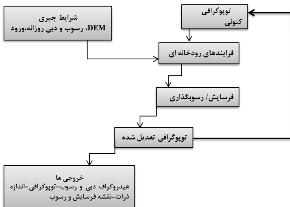
شکل ۲: طرح کلی اجرای مدل سزار (۲۰۰۶, River Basin Dynamics and Hydrology Research Group)
