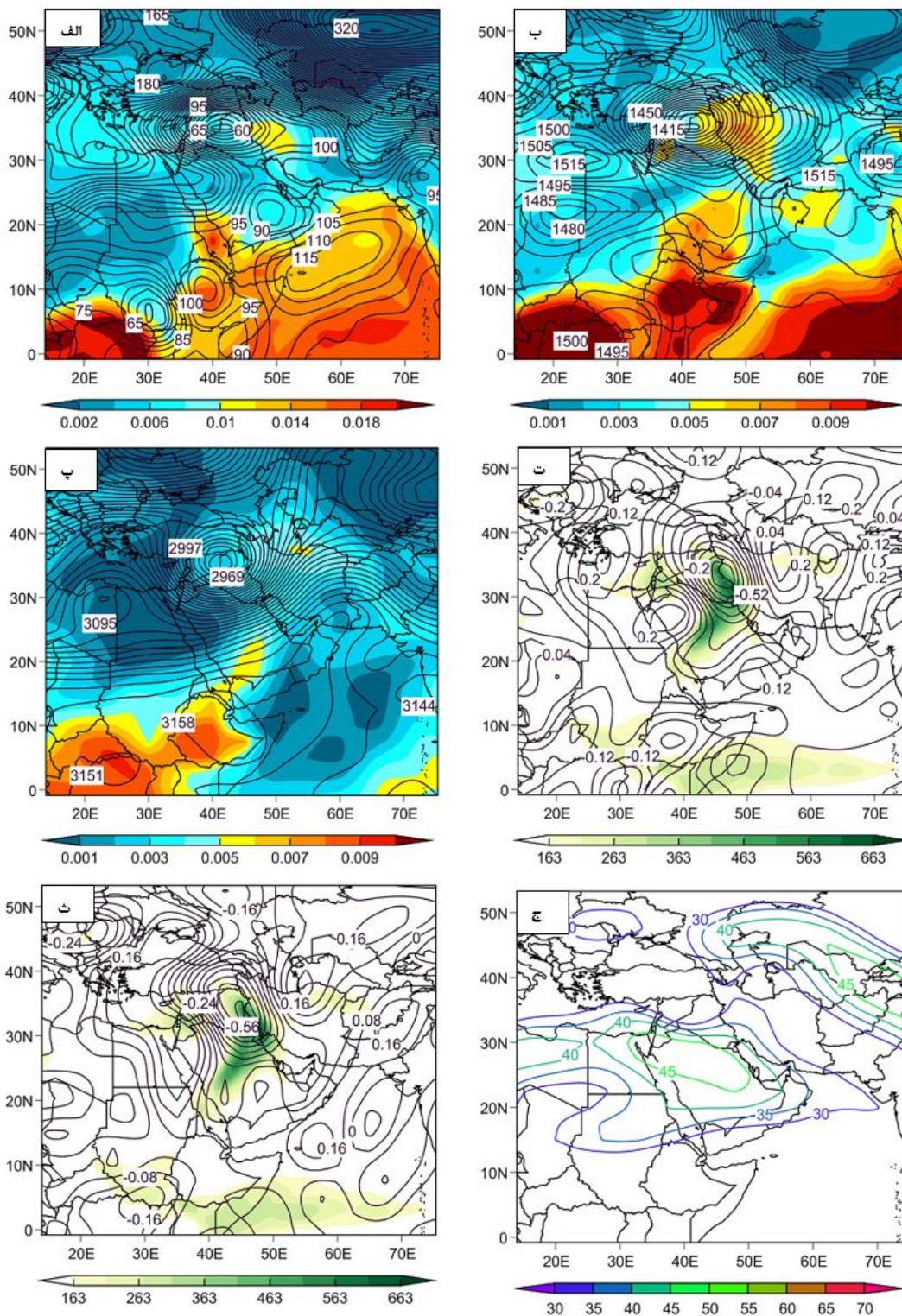
شکل ۱۳. نقشه ترکیبی ژئوپتانسیل متر و نم ویژه به کیلوگرم در کیلوگرم روز ۱۸ فوریه ۲۰۱۸ (تراز ۱۰۰۰، ب) تراز ۸۵۰ و (پ) تراز ۷۰۰ هکتوپاسکال، (ت) نقشه ترکیبی رودخانه (IVT) در ساعت اوج به همراه امگای تراز ۷۰۰ (ت) و تراز ۵۰۰ هکتوپاسکال، (ج) نقشه جت تراز ۲۵۰ هکتوپاسکال
