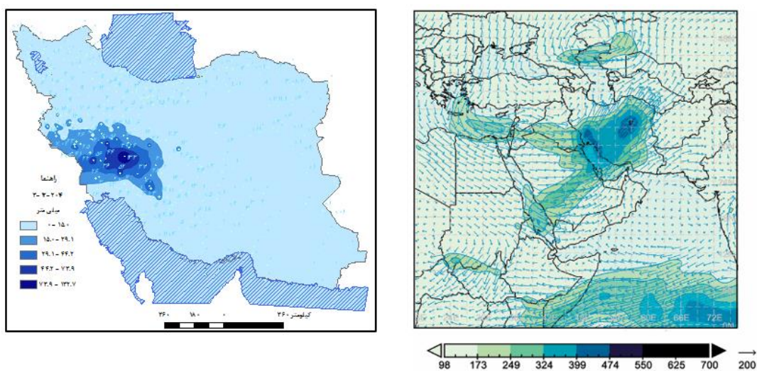
شکل ۱۰. نقشه بارشی روز ۱۲ مارس ۲۰۱۴ (چپ) و نقشه (IVT) رخداد رودخانه جوی در ساعت اوج (راست) با
