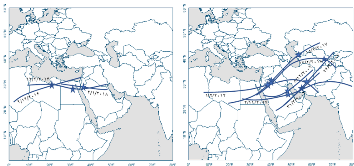
شکل ۱۴. محوهای جت نمونه‌های سودانی (راست) محوهای جت نمونه‌های ادغامی (چپ) در تراز ۲۵۰ هکتوپاسکال
