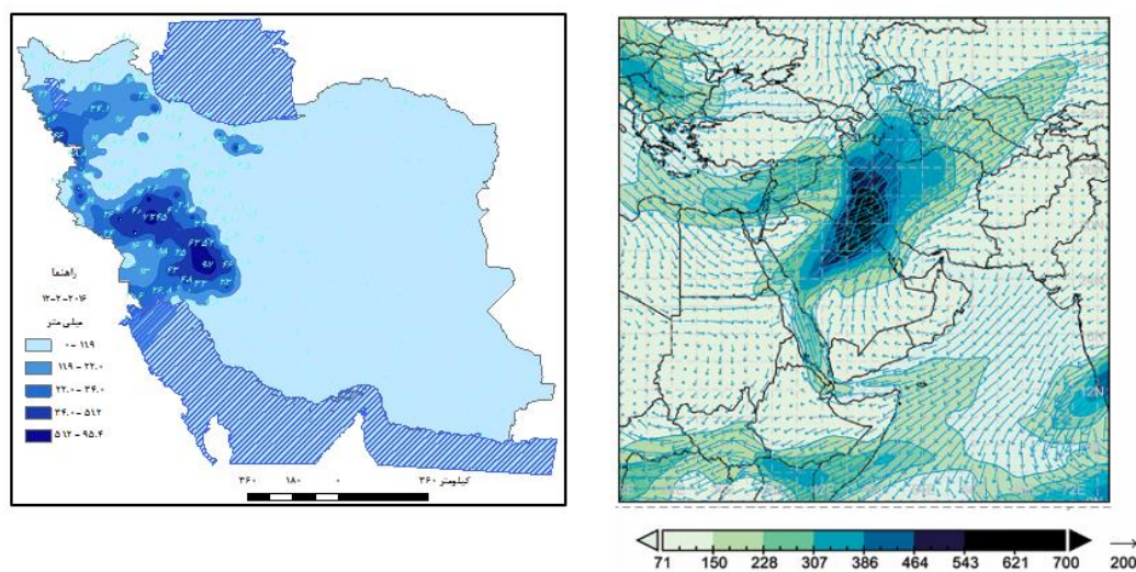
شکل ۱۱. نقشه بارشی روز ۲ دسامبر ۲۰۱۶ (چپ) و نقشه (IVT) رخداد رودخانه جوی در ساعت اوج (راست) با
