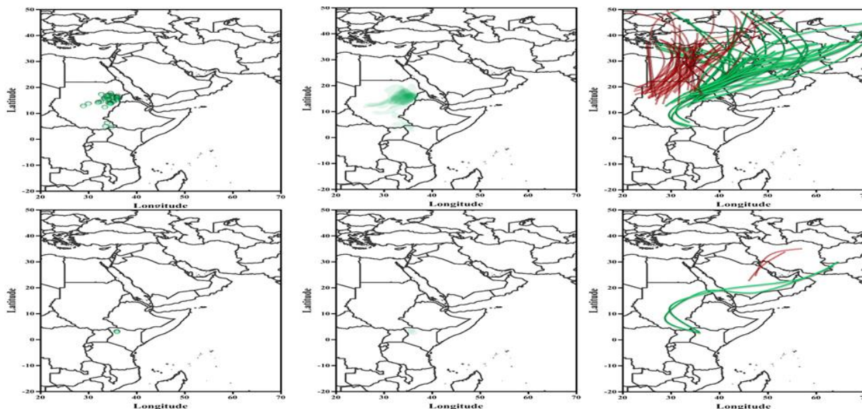
شکل ۴. موقعیت هسته مرکزی (ستون اول) و گسترش اولین منحنی بسته در اطراف هسته مرکزی سامانه کم‌فشار سودان (ستون دوم)، محور گسترش همیدی این سامانه (خطوط سبز) به همراه موقعیت ناوه تراز ۷۰۰ هکتوپاسکال (خطوط قرمز) (ستون سوم) در زمان رخداد بارش‌های جنوب‌غرب (بالا) و جنوب‌میانی (پایین) در ماه اکتبر.
