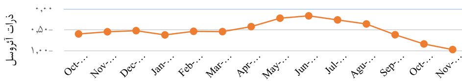
شکل ۵: نمودار تغییرات میانگین ماهانه AI در طول ۲۰۱۸-۲۰۱۹
