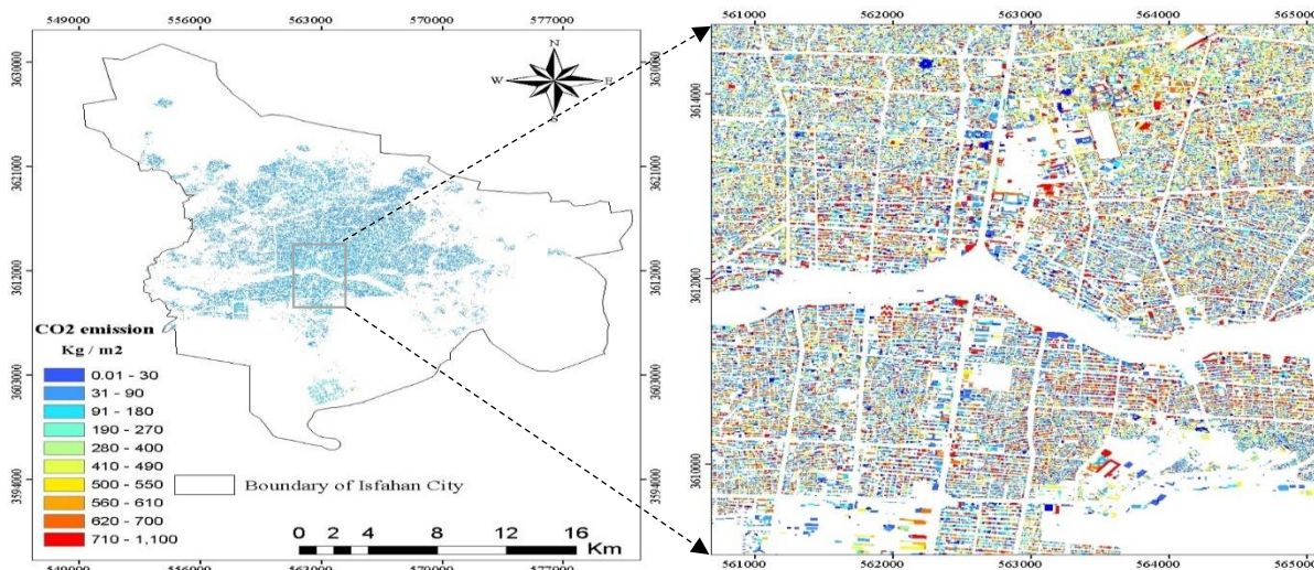
شکل ۲. نقشه توزیع مکانی انتشار سالانه گاز \text{CO}_2 ناشی از احتراق سوخت های فسیلی در بخش خانگی و عمومی -
