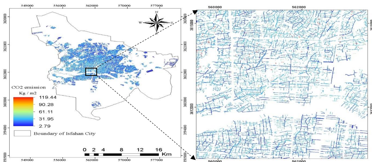
شکل ۵. نقشه توزیع مکانی انتشار سالیانه گاز \text{CO}_2 ناشی از احتراق سوخت های فسیلی از خودروهای سبک در خیابان -
