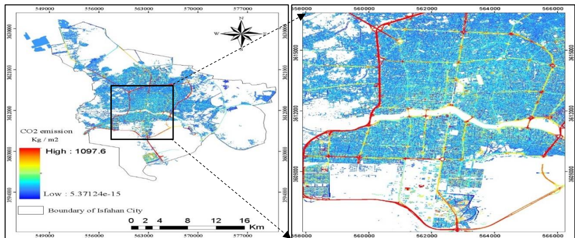
شکل ۸. نقشه توزیع مکانی گاز گلخانه‌ای کربن دی اکسید ناشی از منابع احتراقی ثابت و متحرک (بخش خانگی، تجاری -
