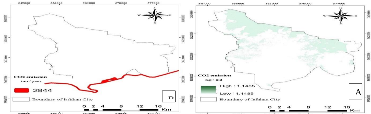
شکل ۷. نقشه مکانی انتشار سالیانه گاز CO 2 ناشی از احتراق سوخت‌های فسیلی در اراضی کشاورزی (A) و حمل و نقل
