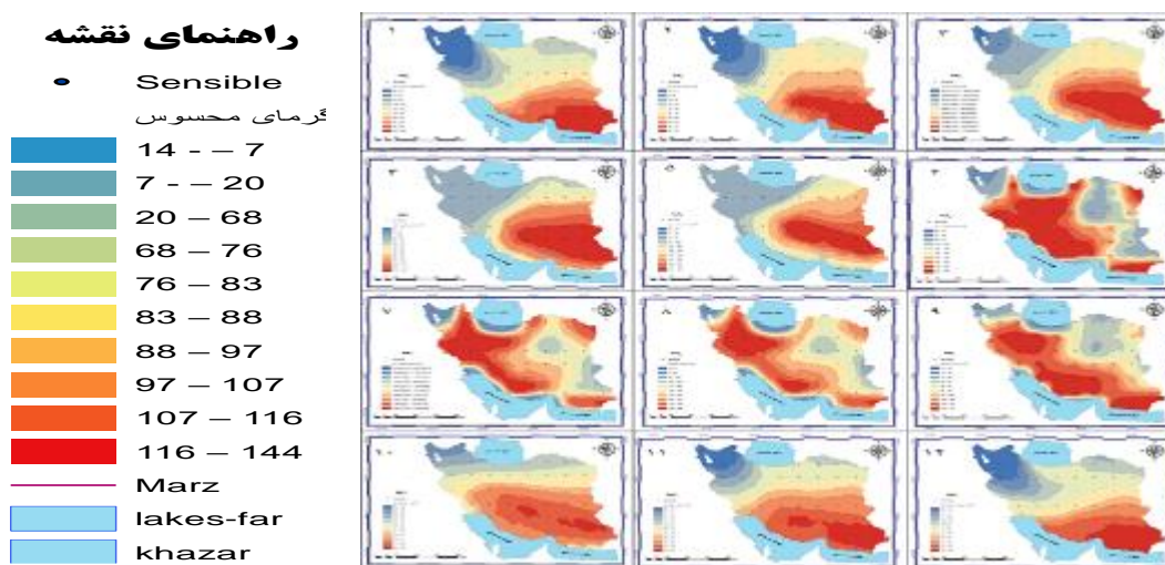
شکل ۳. نقشه های ماهانه شار گرمای محسوس دوره مطالعاتی (۱۹۴۸-۲۰۲۰). به ترتیب شماره ۱ ماه ژانویه و ۱۲ ماه دسامبر
