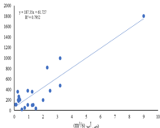
شکل ۸. منحنی سنج رسوب ایستگاه سفیدچاه (فصل تابستان)
