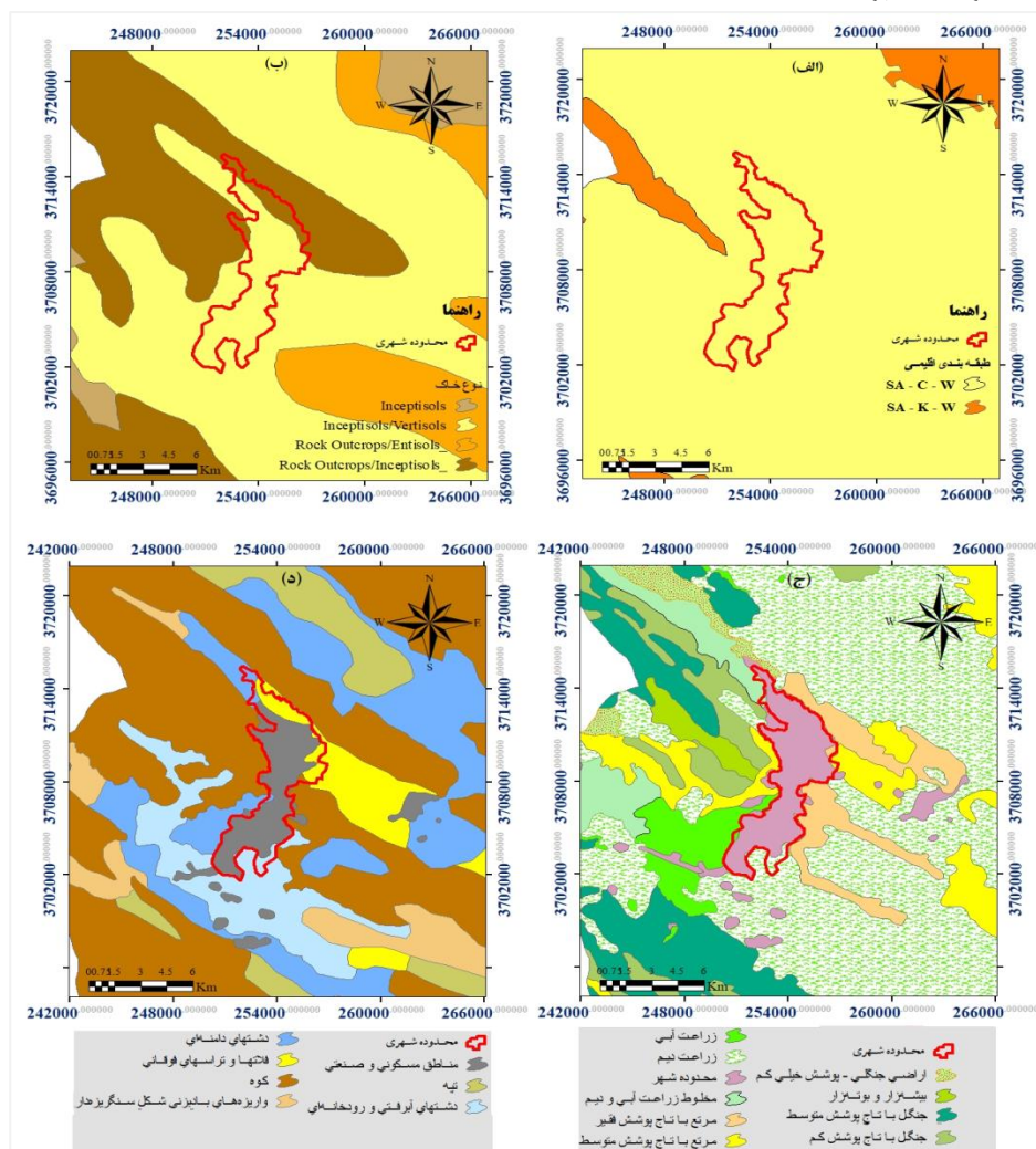
شکل ۷. مؤلفه های تأثیر گذار بر تغییر پذیری زیستگاه های منطقه
