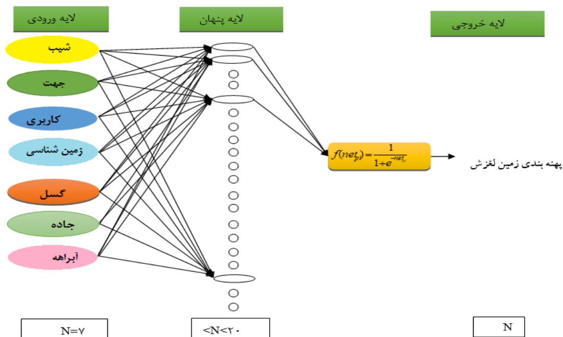
شکل ۲. ساختار شبکه عصبی مصنوعی به کار رفته در حوضه آبخیز میسخاص
