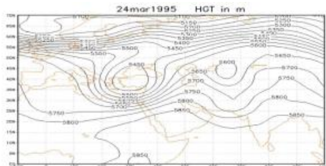
شکل ۱۶: نقشه ارتفاع ژئوپتانسیل در تراز ۵۰۰ هکتوپاسکال در روز ۲۴ مارس ۱۹۹۵
