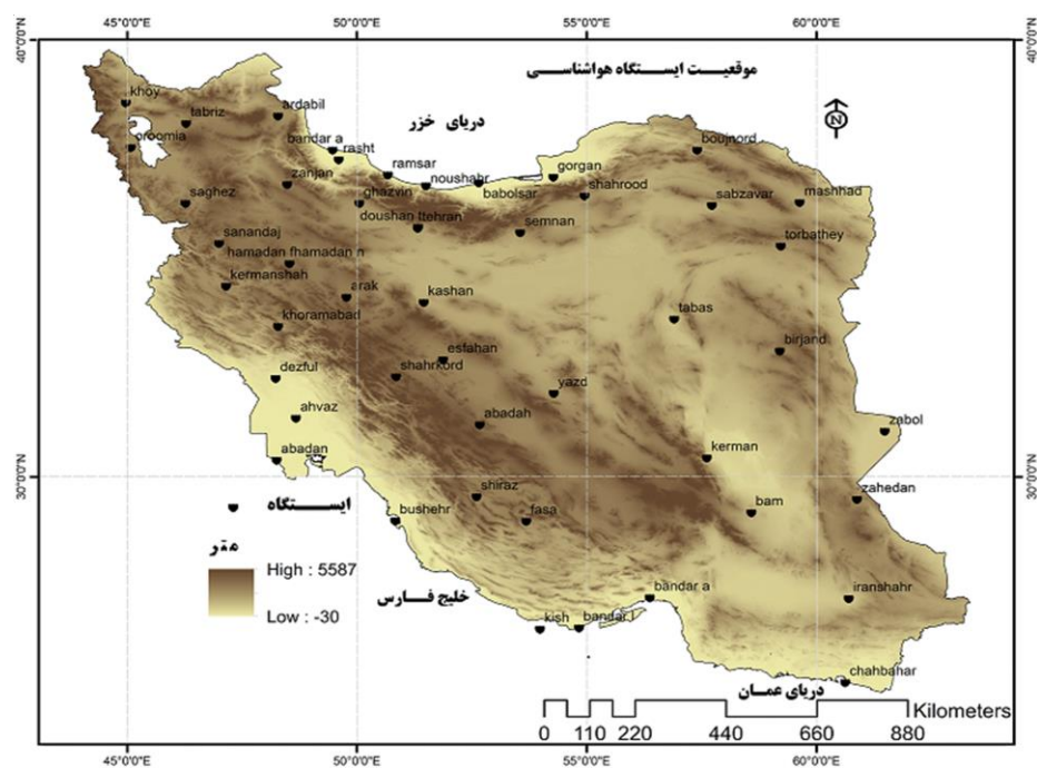
شکل ۱: موقعیت ایستگاههای سینوپتیک روی فلات ایران.
