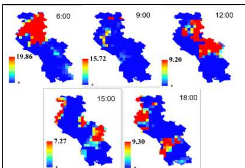
شکل ۱۴: بارش (میلیمتر در ساعت) در طی ساعتهای مختلف با استفاده از نتایج محصول ساعتی ۳B۴۲ ماهواره TRMM در روز ۲۹ اکتبر ۲۰۱۵.
