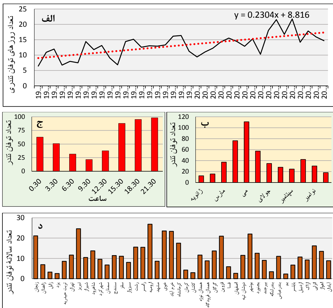
شکل ۲: الف: میانگین سالانه تعداد توفان‌های تندری در ایران به‌همراه شیب خط رگرسیون و ناهنجاری طی دوره آماری (۲۰۱۶-۱۹۸۰)؛ ب: میانگین ماهانه تعداد توفان‌های تندری طی دوره آماری (۱۹۸۰-۲۰۱۶)؛ ج: میانگین ساعتی تعداد توفان‌های تندری طی دوره آماری (۲۰۱۶-۱۹۸۰)؛ د: میانگین سالانه تعداد توفان‌های تندری طی دوره آماری (۲۰۱۶-۱۹۸۰)
