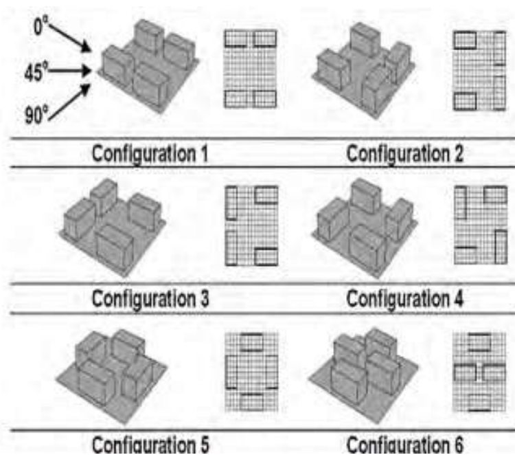
شکل ۸: تغییر شرایط آسایش اقلیمی پیرامونی ساختمان‌های بلند از طریق تغییر ساختار مجموعه و موقعیت ساختمان‌ها نسبت به یکدیگر منبع: (Hong & Lin, ۲۰۱۵)
