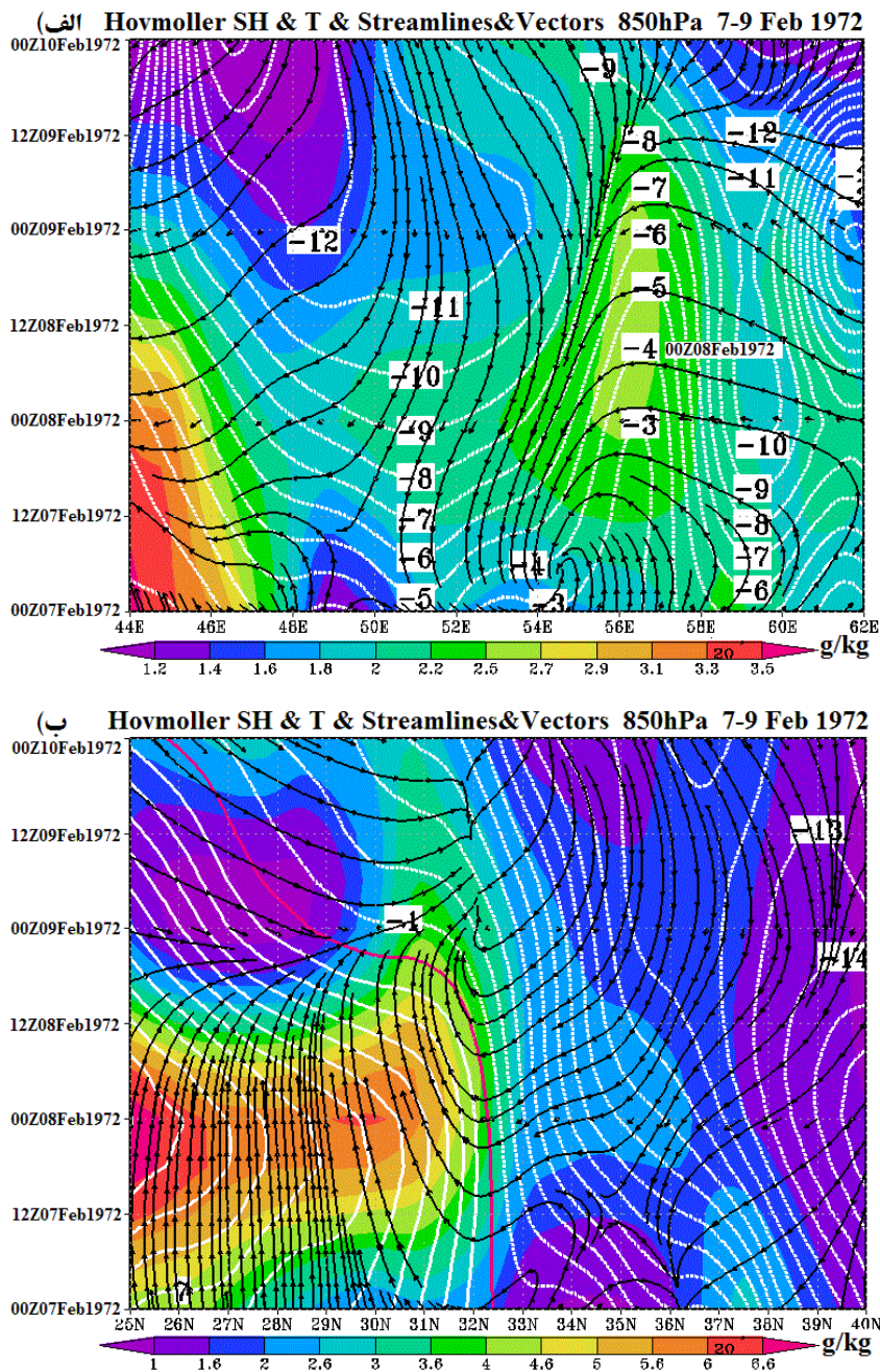
شکل ۴. نمودارهای نیمرخ قائم رطوبت و ویژه (سایه روشن)، دما (پررنگ‌های سفیدرنگ) و جریان باد (پیکان‌های سیاه‌رنگ) تراز ۸۵۰ هکتوپاسکال برای طول جغرافیایی ۵۰ درجه شرقی (الف) و عرض جغرافیایی ۳۶ درجه شمالی (ب) برای دوره رخداد فرین برفی ۷-۹ فوریه ۱۹۷۲ در ایران.
