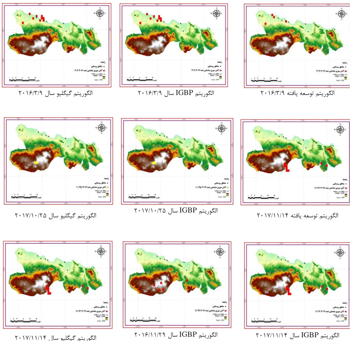
شکل ۳. نقشه آتش سوزی های شناسایی شده الگوریتم های شناسایی آتش سوزی پناهگاه حیات وحش کیامکی داغ
