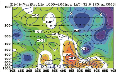
شکل ۱۶. نیمرخ قائم تاوایی و واگرایی برای عرض ۳۲ درجه (عرض شهر اصفهان) (الگوی اول)
