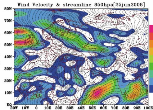
شکل ۲۴. جریان و سرعت باد د تراز ۸۵۰ هکتوپاسکال(الگوی اول)
