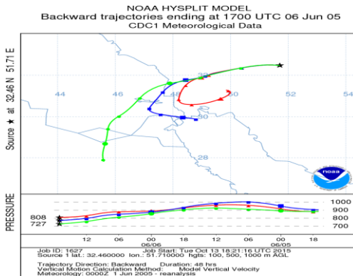
شکل ۲۲. ردیابی ذرات معلق به روش پسگرد(الگوی سوم) شکل ۲۳. ردیابی ذرات معلق به روش پسگرد(الگوی چهارم)
