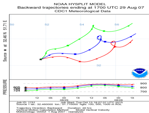
شکل ۲۰. ردیابی ذرات معلق به روش پسگرد(الگوی اول) شکل ۲۱. ردیابی ذرات معلق به روش پسگرد(الگوی دوم)
