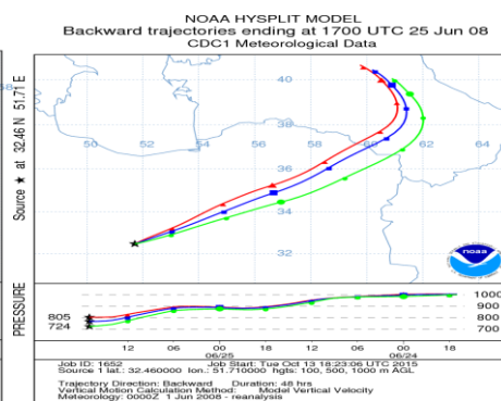
شکل ۲۰. ردیابی ذرات معلق به روش پسگرد(الگوی اول)
