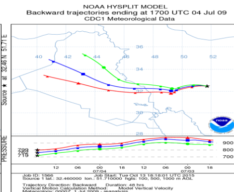
شکل ۲۲. ردیابی ذرات معلق به روش پسگرد(الگوی سوم)
