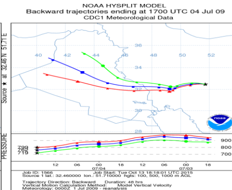
شکل ۲۲. ردیابی ذرات معلق به روش پسگرد(الگوی سوم) شکل ۲۳. ردیابی ذرات معلق به روش پسگرد(الگوی چهارم)
