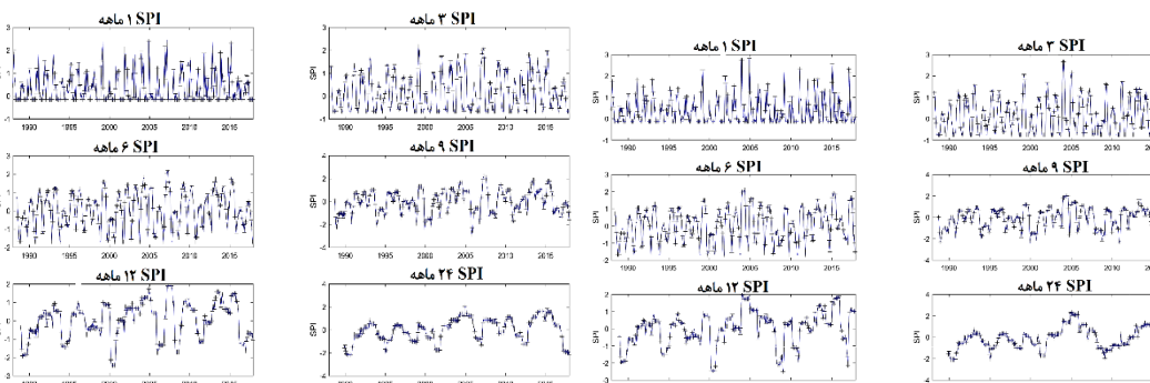
شکل ۶. SPI ایستگاه مروست
