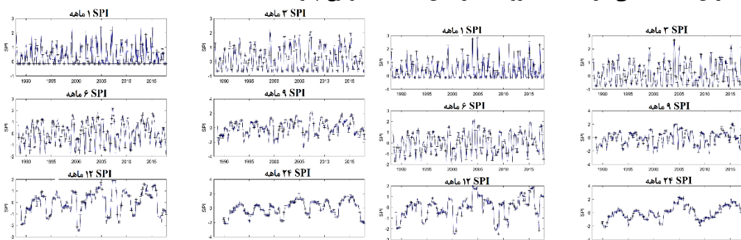
شکل ۶. SPI ایستگاه مروست
