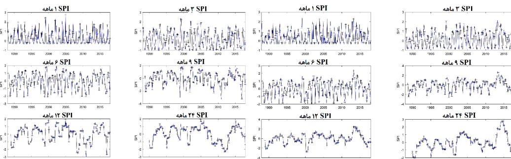
شکل ۴. SPI ایستگاه یزد
