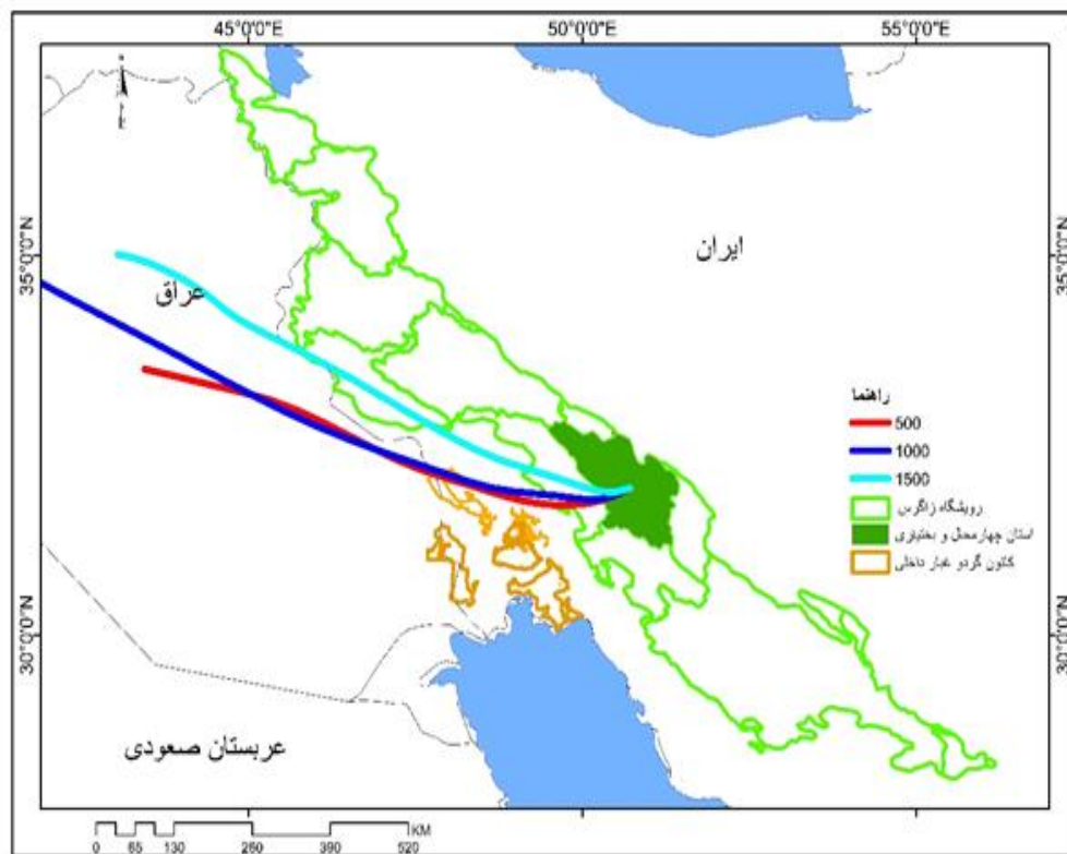
شکل ۱۱- منشاء و مسیر ورود ذرات گرد و غبار به جنگل‌های زاگرس استان چهارمحال و بختیاری از سمت شمال غرب ۰۵/۰۷/۲۰۰۹
