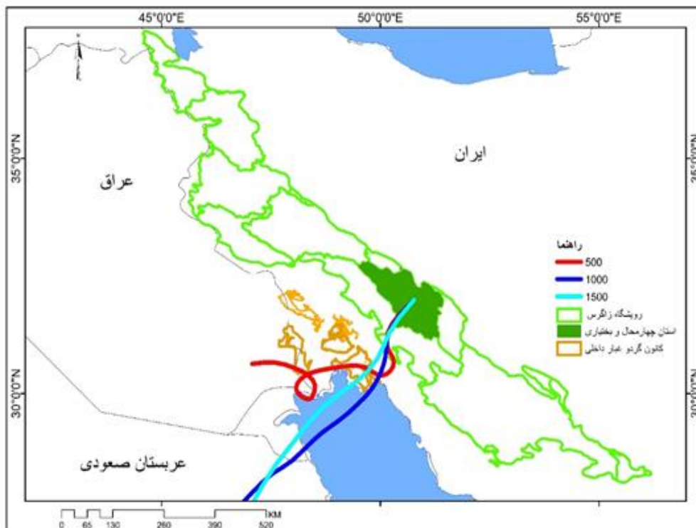
شکل ۱۰- منشاء و مسیر ورود ذرات گرد و غبار به جنگل‌های زاگرس استان چهارمحال و بختیاری از سمت جنوب غرب ۲۳/۰۵/۲۰۱۲
