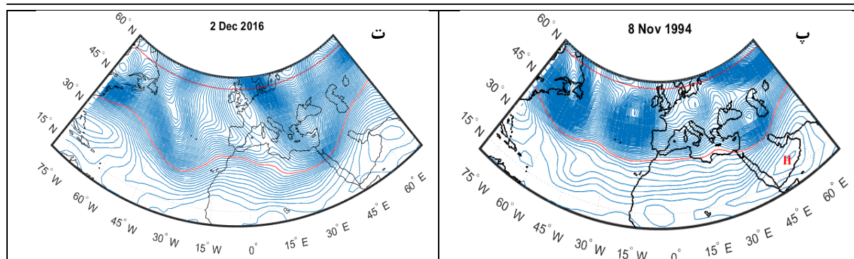
شکل ۱۲. الگوی تموج تراز ۵۰۰ هکتویاسکال برای فوریه ۱۹۹۳ (الف)، مارس ۲۰۱۹ (ب)، نوامبر ۱۹۹۴ (پ) و دسامبر ۲۰۱۶ (ت)
