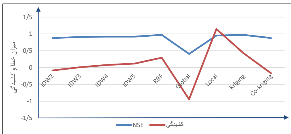
شکل شماره ۷) نمودار خطی میزان خطای NSE و میزان کشیدگی روش‌های درونیابی
