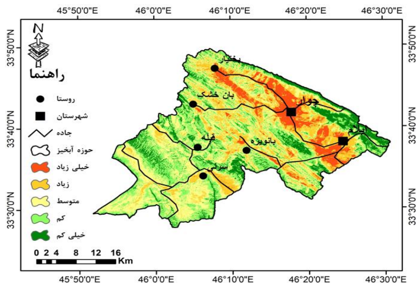
شکل ۶ نقشه طبقات پهنه‌بندی حساسیت فرسایش گالی با استفاده از مدل دمستر-شفر
