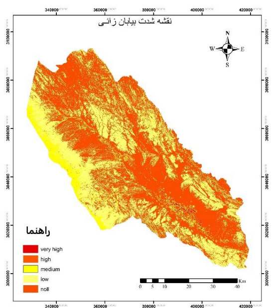
شکل (۵). نقشه شدت بیابان‌زایی حاصل از معادله I = a * NDVI - Albedo
