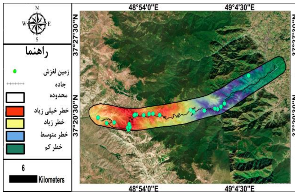
شکل ۱۷. نقشه پهنه بندی خطر وقوع زمین لغزش در جاده ماسال به گیوان
