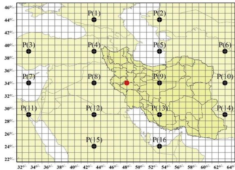
شکل ۲. مختصات ۱۶ نقطه اطراف نقطه مرجع به روش لمب_جنکینسون در محدوده مورد مطالعه
