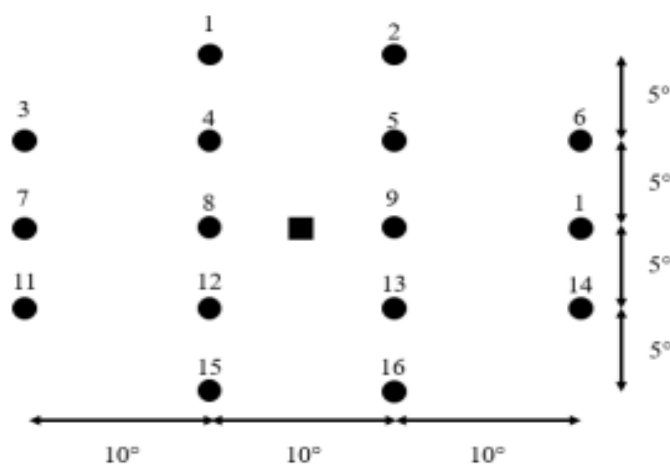
شکل ۱. توزیع فضایی ۱۶ نقطه روش لمب_جنکینسون. مربع نشان دهنده مرکز شبکه می‌باشد (لای ۲ ، ۲۰۱۰).
