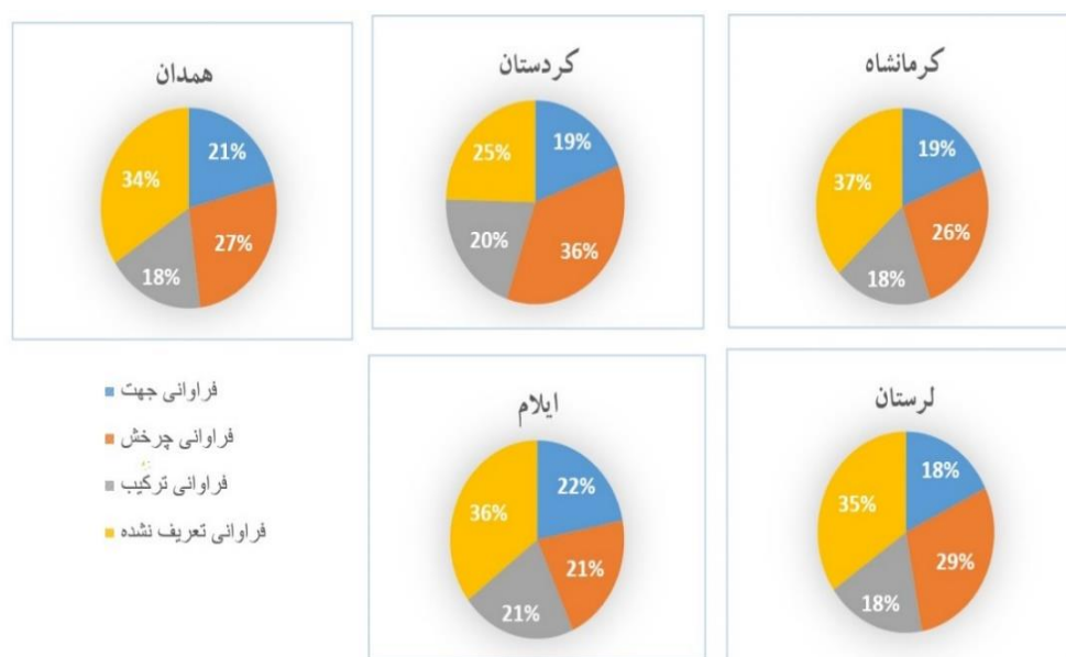
شکل ۸. درصد فراوانی رخداد هریک از حالت‌های مربوط به روش L-J برای ۵ استان
