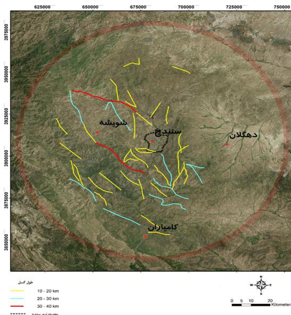
شکل ۲. توزیع گسل‌های با طول بیش از ۱۰ کیلومتری واقع در شعاع ۷۰ کیلومتری سنج
