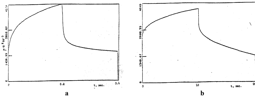
شکل ۴- (a) منحنی کروموتولومتری الکتروده نازک طلا 300 \text{ \AA} در الکترولیت 0.1 \text{ mol LiClO}_4 ، تغییرات پتانسیل از 0.5 به 0.35 ولت نسبت به SCE (b) منحنی کروموتولومتری الکتروده نازک ( 1000 \text{ \AA} ZnPC) در الکترولیت 0.1 \text{ mol LiClO}_4 ، تغییرات پتانسیل از 0.5 به 0.35 ولت نسبت به SCE
